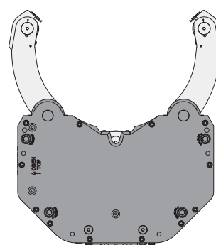
RX 6 Spannbereich 100 - 520 mm
