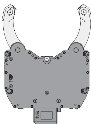
K 6.1 Spannbereich 215 - 510 mm
