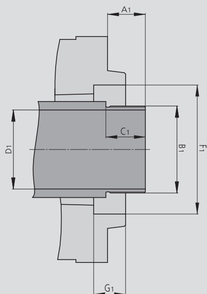
Naso macchina con attacco ISO/cono corto
