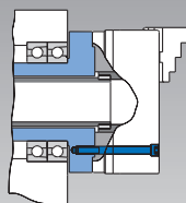
Centrajes normalizados según DIN 55026
