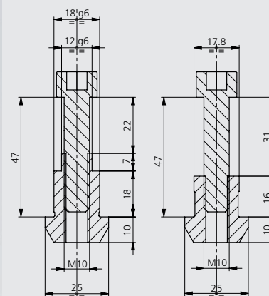
► T-SLOT 18 46204102
