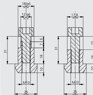
► T-SLOT 18 46204105
