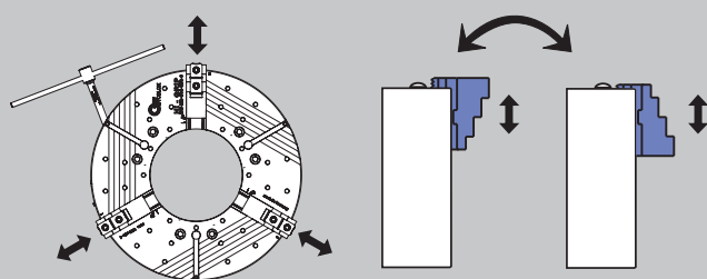
Garras ajustables radialmente
